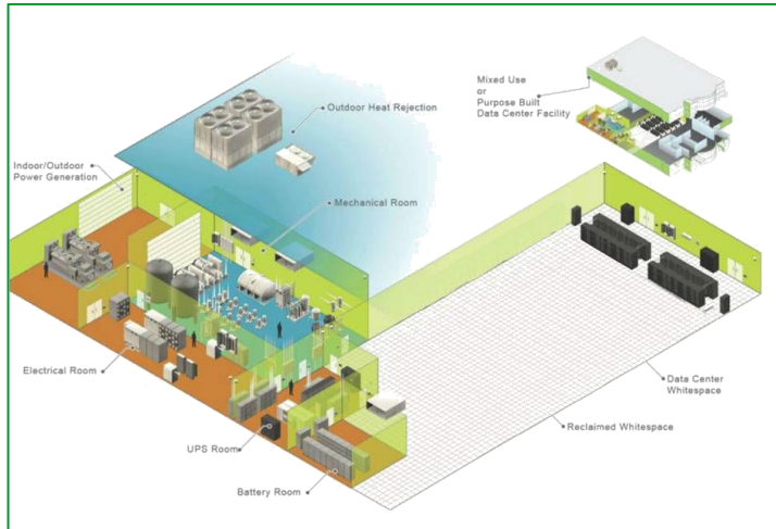
Vue 3D du datacenter conventionnel
