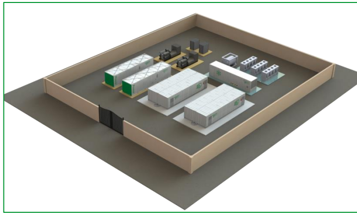
Vue 3D du datacenter conventionnel
