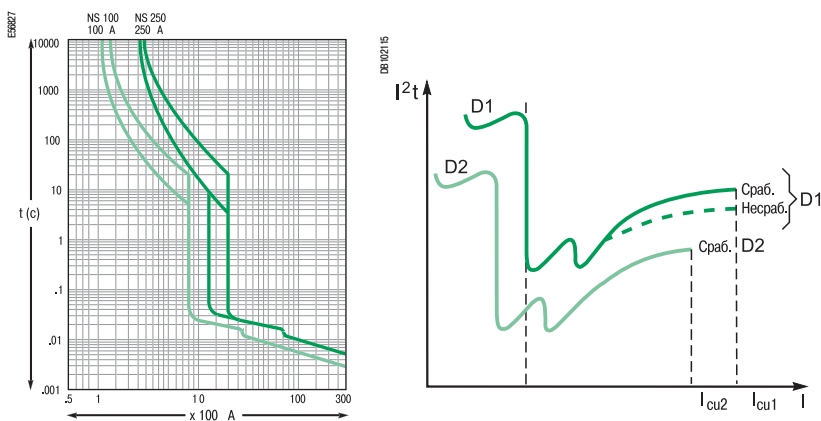
Время-токовые характеристики и кривые энергии аппаратов Compact NSX 100 и 250 A.
