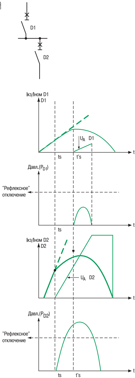
Селективность, усиленная каскадным соединением: описание принципа
