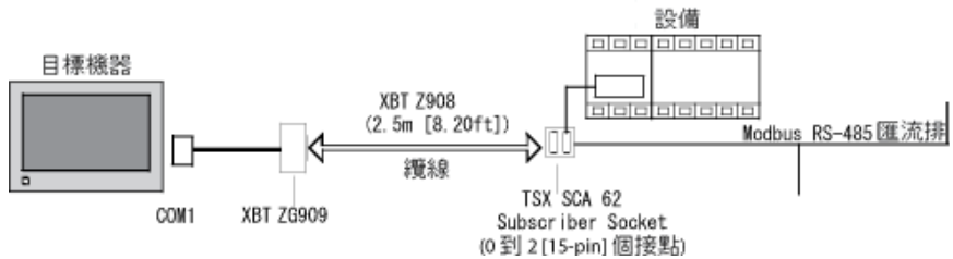
圖 16 HMIGTO 系列 (不包含 HMIGTO1310)、iPC 系列、XBT GK 系列、XBT GT2000 系列或以上、XBT GTW 系列、XBT GC 2000 系列
