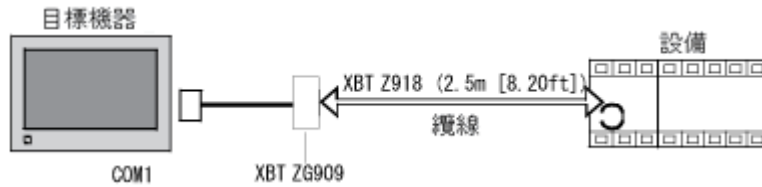
圖 15 XBT GT 2000 系列或以上、XBT GK 系列、XBT GC 2000 系列
