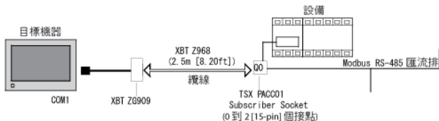
圖 19 XBT GK 系列、XBT GK 系列、HMIGTO 系列、HMISTO 系列、HMISTU 系列
