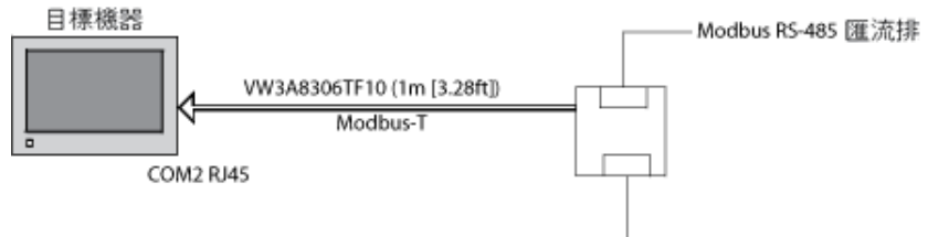
圖 5 XBT GK 系列、XBT GK 系列、HMIGTO 系列、HMISTO 系列、HMISTU 系列 RS 485
