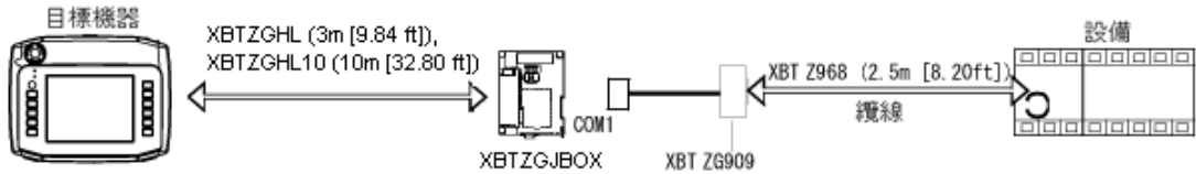
圖 24 XBT GH 2000 系列
