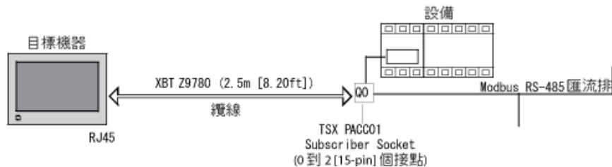
圖 18 XBT GT 2000 系列或以上、XBT GK 系列、XBT GC 2000 系列
