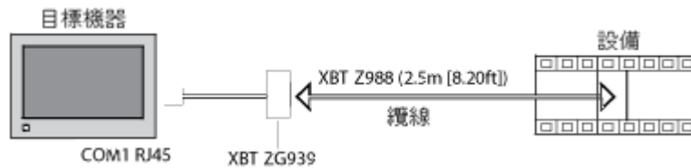
圖 9 XBT GT1000 系列、XBT GT1005 系列、HMIGTO1310、HMISTO 系列、HMISTU 系列 RS 232C
