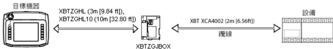
圖 32 XBT GH 2000 系列
