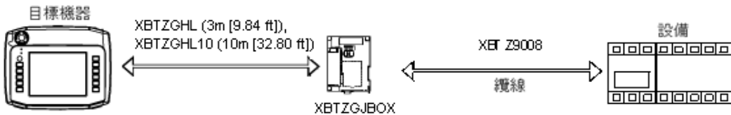
圖 30 XBT GH 2000 系列
