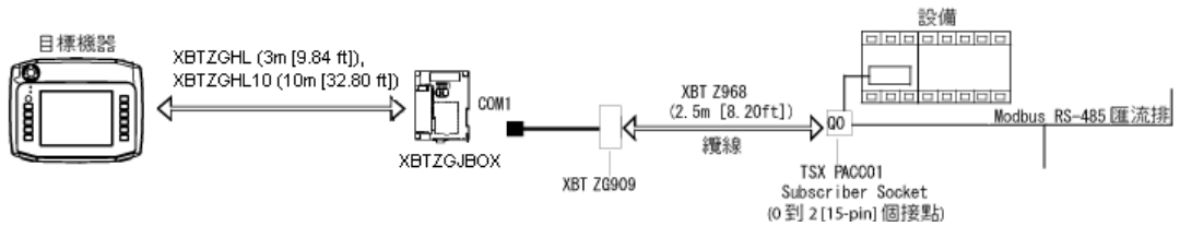
圖 25 XBT GH 2000 系列
