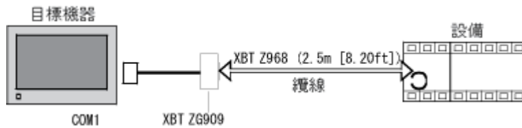
圖 10 XBT GT 2000 系列或以上、XBT GK 系列、XBT GC 2000 系列 RS 485
