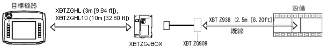
圖 29 XBT GH 2000 系列
