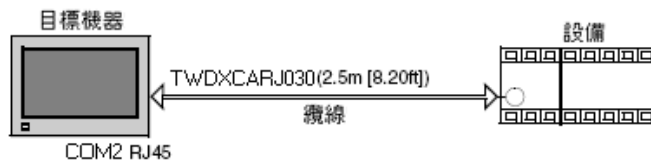
圖 22 XBT GK 系列、XBT GT 系列、HMIGTO 系列、HMISTO 系列、HMISTU 系列
