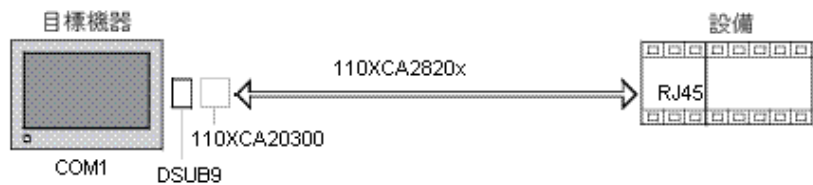
圖 33 HMIGTO 系列 (不包含 HMIGTO1310)、iPC 系列、XBT GTW 系列、XBT GC2000 系列、XBT GK 系列、XBT GT 2000 系列或以上
