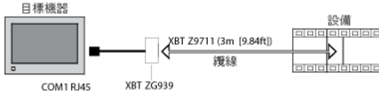
圖 8 XBT GT1000 系列、XBT GT1005 系列、HMIGTO1310、HMISTO 系列、HMISTU 系列 RS 232C
