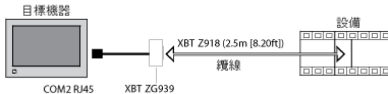
圖 6 XBT GK 系列、XBT GK 系列、HMIGTO 系列、HMISTO 系列、HMISTU 系列 RS 485
