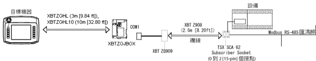
圖 33 HMIGTO 系列 (不包含 HMIGTO1310)、iPC 系列、XBT GTW 系列、XBT GC2000 系列、XBT GK 系列、XBT GT 2000 系列或以上
