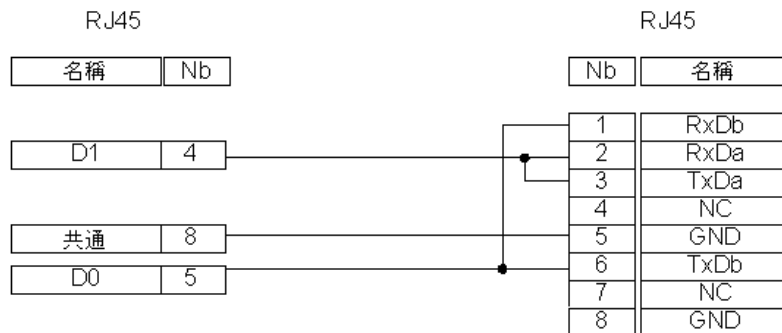
圖 36 XBT GT 1000 系列、XBT GT 1005 系列、HMIGTO 系列、HMISTO 系列、XBT GK 系列、XBT GT 2000 系列或以上
