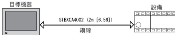
圖 16 HMIGTO 系列 (不包含 HMIGTO1310)、iPC 系列、XBT GK 系列、XBT GT2000 系列或以上、XBT GTW 系列、XBT GC 2000 系列
