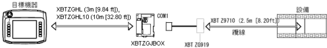
圖 26 XBT GH 2000 系列
