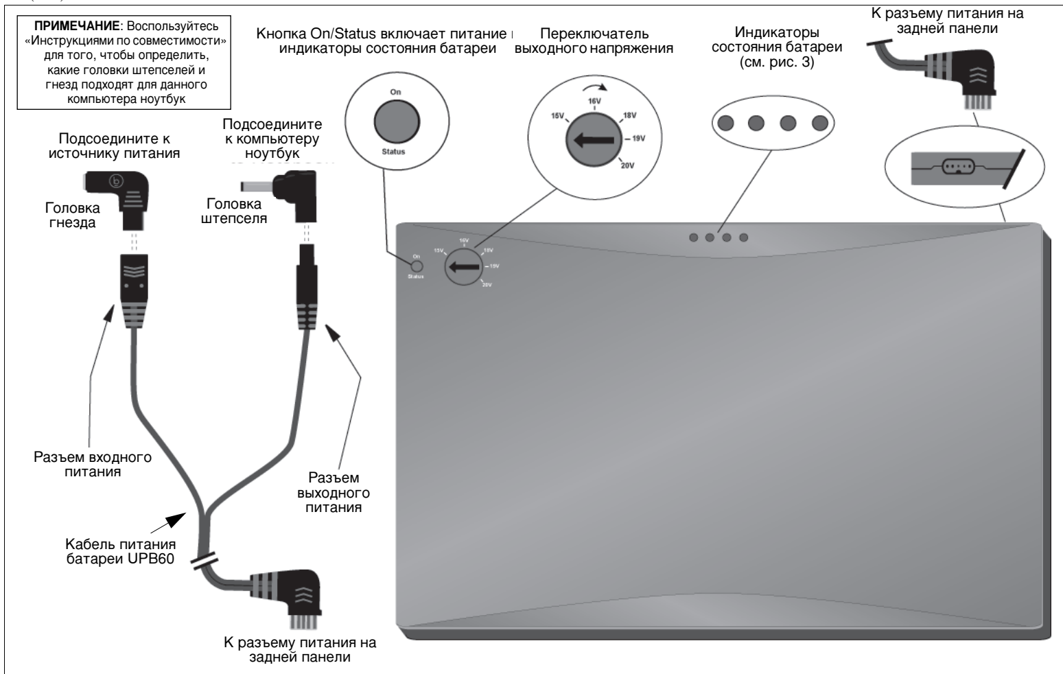
Рисунок 1. Пользовательский интерфейс Универсальной батареи UPB60 для портативных компьютеров ноутбук
