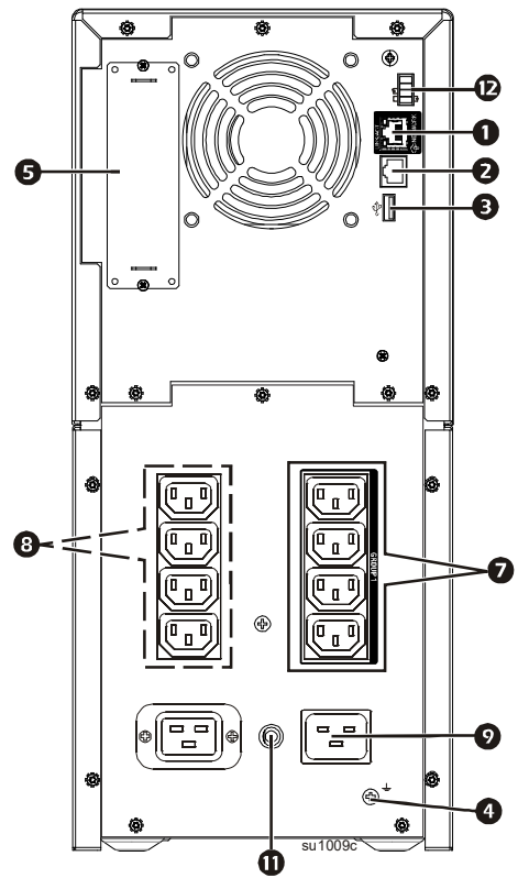
SMT2200IC и SMT3000IC вертикальный корпус
