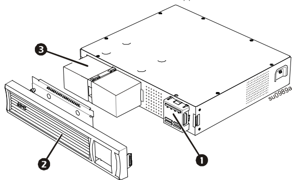
SMT1000RM2UC, SMT1000RM12UC, SMT1500RM2UC и SMT1500RM12UC для монтажа в стойку
