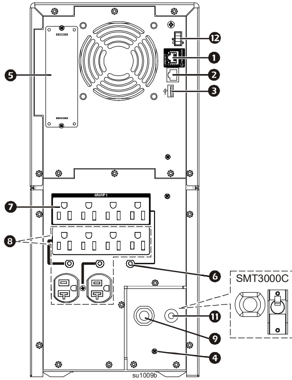
SMT2200C и SMT3000C вертикальный корпус
