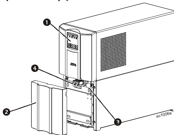
SMT2200C, SMT2200IC, SMT3000C и SMT3000IC вертикальный корпус
