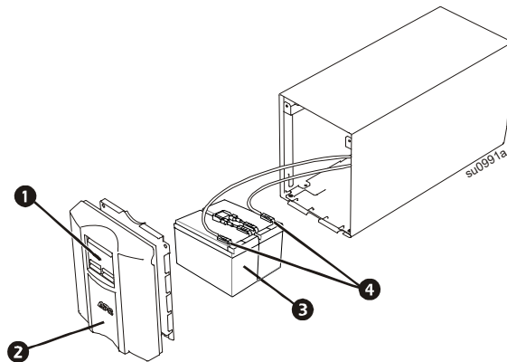
SMT2200C, SMT2200IC, SMT3000C и SMT3000IC вертикальный корпус
