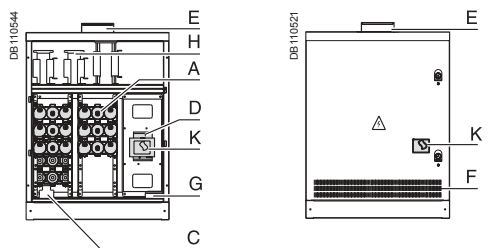
Fig. 6 : armoire A2.
