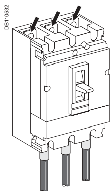
Fig. 10 : raccordement de puissance sur disjoncteur.
