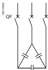
Fig. 1 : schémas électriques de principe, type Varsset Direct et Varsset Direct avec disjoncteur.
