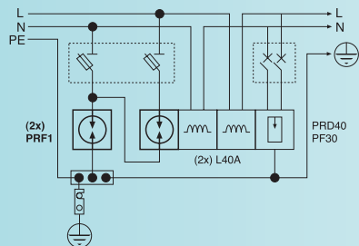
TN-S - 1P+N - MC/MD
