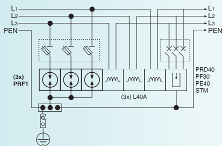
TN-C - 3P - MC
