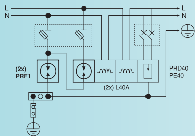
TT - 1P+N - MC/MD
