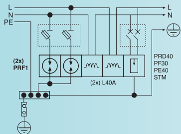
TN-S - 1P+N - MC
