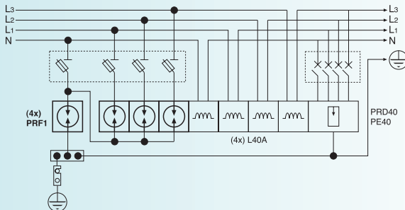
TN-S - 3P+N - MC
