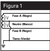
Figura 1 FASE DIVIDIDA 2 fases, 1 neutro 1 tierra
