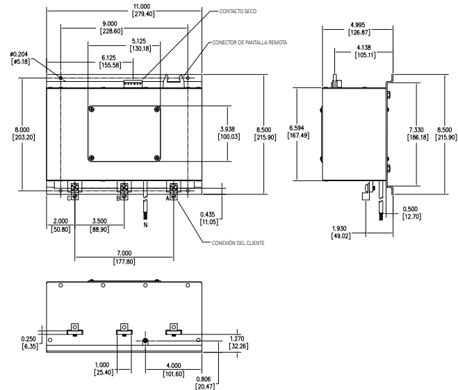
Figura 3 TRIÁNGULO FASE ALTA (B Alta) trifásico, (B Alta), 1 neutro, 1 tierra
