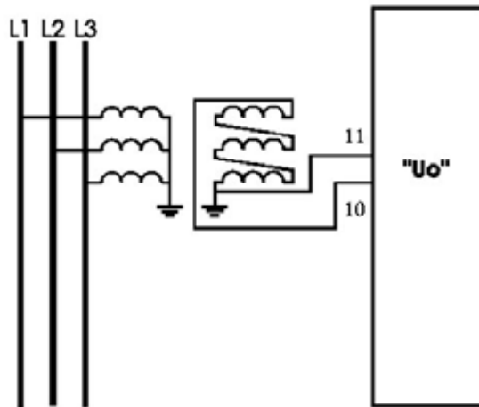
Рис. 5.9-1 Схема "разомкнутый треугольник" в режиме измерения "Uo"
