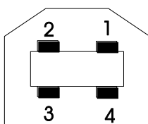
Рис. 9.3.1-1 Нумерация контактов на передней панели USB контактора типа В
