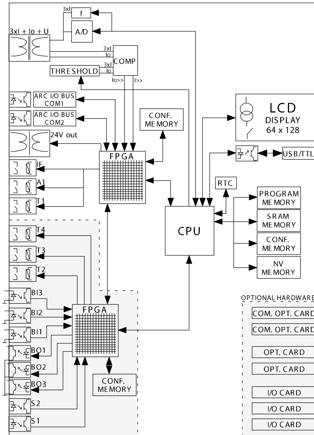
Рис. 9.4.1-1 Функциональная блок-схема для VAMP 321 АВ ААА ААААА А1
