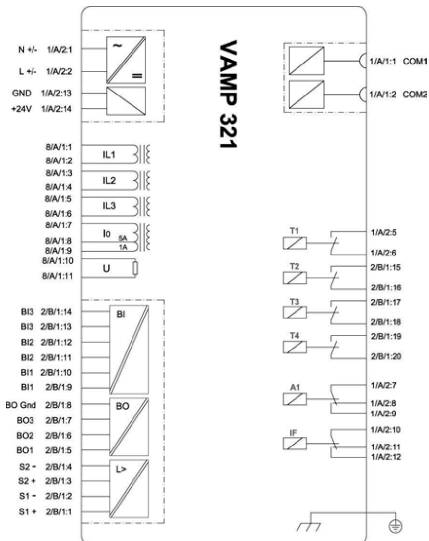
Рис. 9.4.2-1 Функциональная блок-схема для VAMP 321-АВААА-ААААА-А1/2/3
