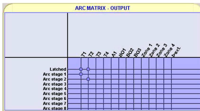
Рис. 3.1.3-5 Пример настройки матрицы выходных сигналов
