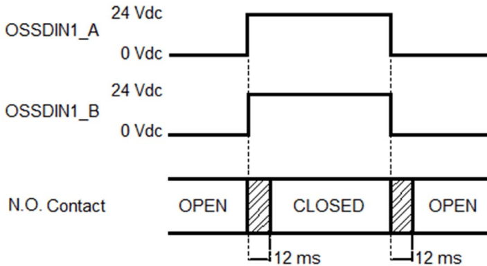
Diagrama de temporização
