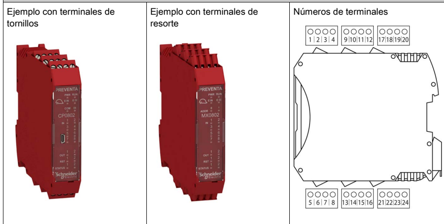
Módulo XPSMCMER0002•
