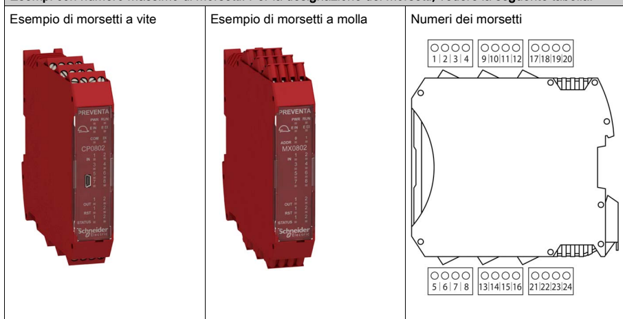
Modulo XPSMCMER0002•
