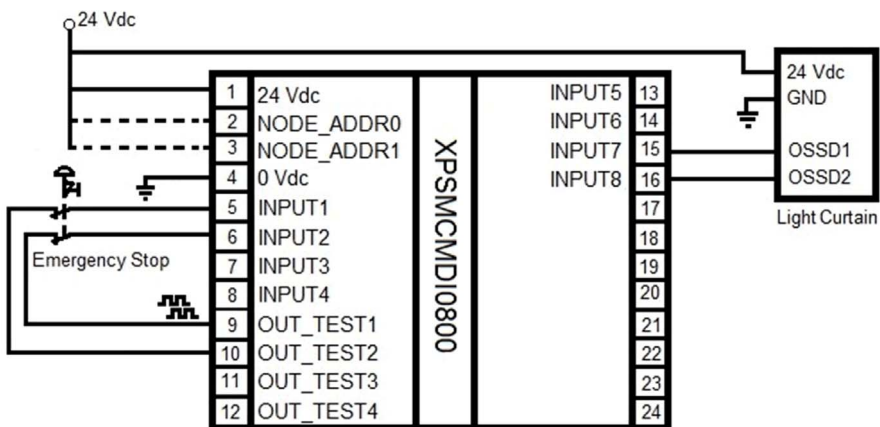
XPSMCMDI0800• 模块
