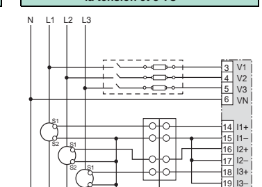
Figure 8 : Raccordement triphasé en étoile en 4 fils, avec raccordement direct de la tension et 3 TC
