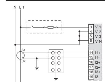
Figure 3 : Réseau monophasé phase-neutre 2 fils 1 TC
