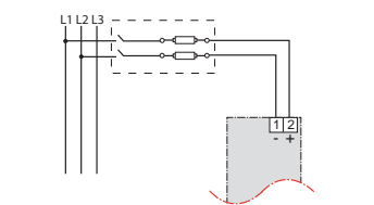
Figure 21 : Alimentation par raccordement direct (entre phases)
