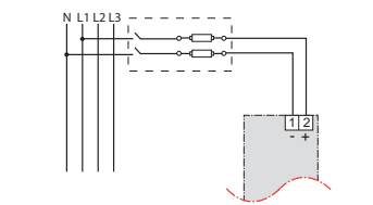
Figure 22 : Alimentation par raccordement direct (phase-neutre)
