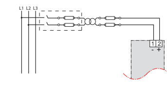
Figure 24 : Raccordement à un transformateur d'alimentation (TA)
