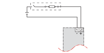
Figure 23 : Alimentation par raccordement direct (alimentation en courant continu)
