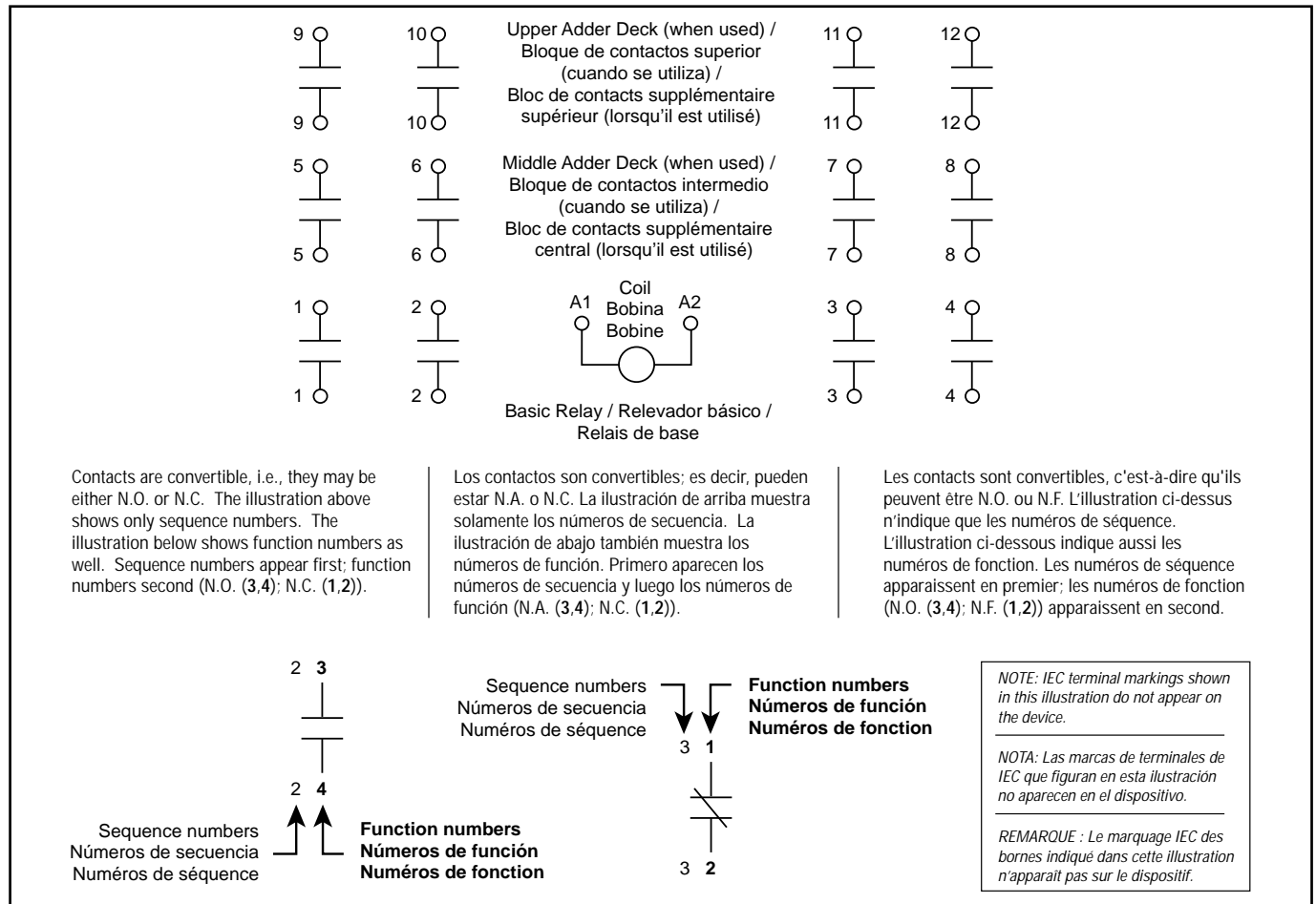
Figure / Figura / Figure 2 : Wiring Diagram / Diagrama de cableado / Schéma de câblage
