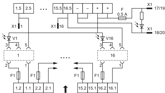
ABE-6S16E
