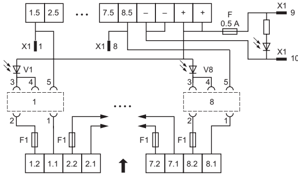
ABE-6S16E
