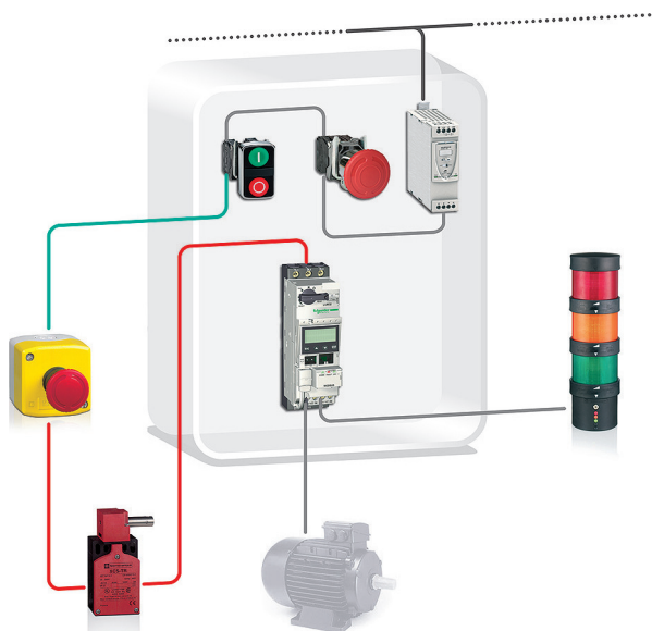
Zwolnienie momentu silnika (Power Removal, PL c, SIL 1)
