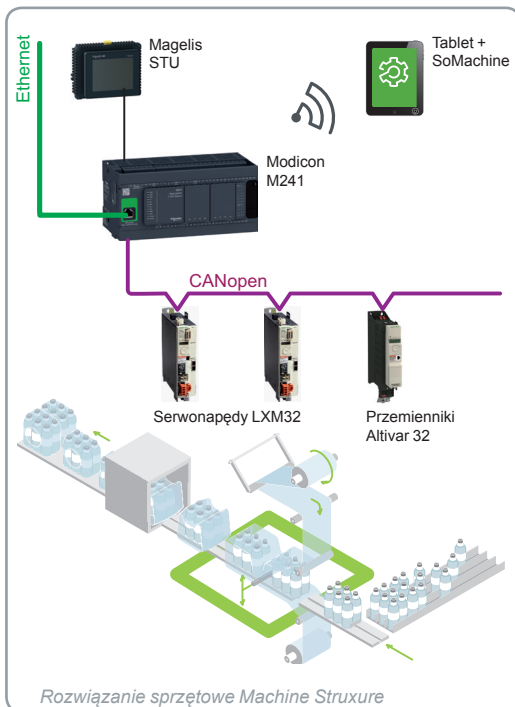
Rozwiązanie sprzętowe Machine Struxure
