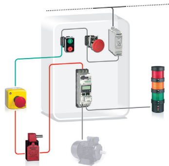
Bezpieczny STOP 0 (PL d, SIL 2)
