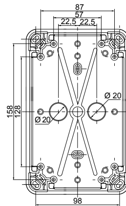
Rückseite
