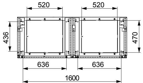
Schrankbreite 1600 mm
