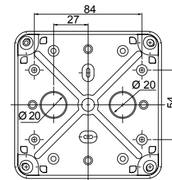
Rückseite
