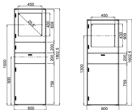
PC-Modulträger mit einer Höhe von 1800 mm.
