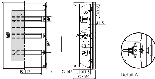
Ausschnitt Frontplatte
