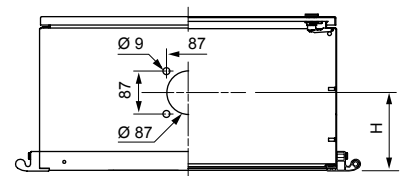
Abb. 2 Schranktiefe 300
