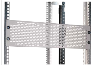
19" Abdeckplatten mit Lüftungsschlitzen Stahl: 1,5 mm
