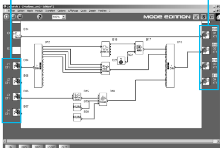
Fenêtre d'Edition de programme FBD
