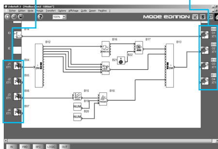
Fenêtre d'Édition de programme FBD
