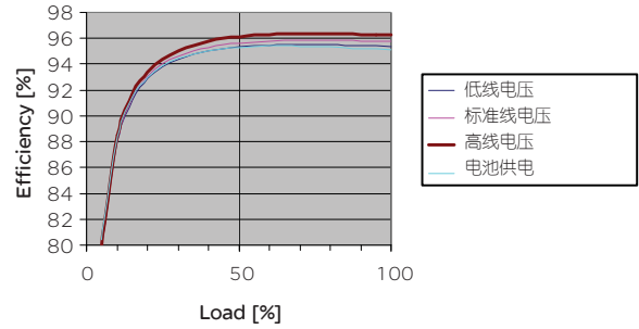
Galaxy 3500系列30kVA 效率曲线
