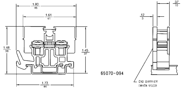
Type GP6
