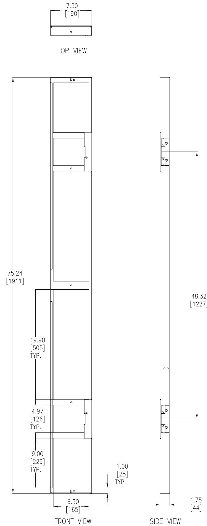
RIGHT SIDE PLENUM
