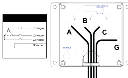
Figura 10: Instalación en delta de tres fases, 3 hilos
