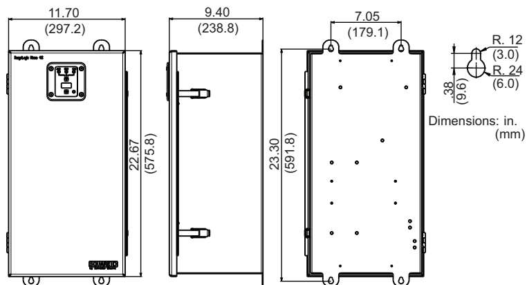
Figure 6: Gabinetes NEMA 4X de 11 x 23 pulg con o sin opción de interruptor integral/SWT
