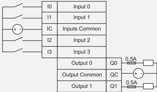
Verdrahtung des digitalen E/A
