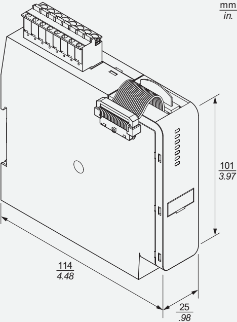
Digitales E/A-Modul: TPRDG4X2
