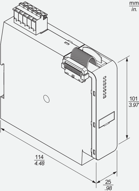
SIL-Schnittstellenmodul: TPRSM001
