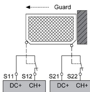
Schutztürüberwachung
