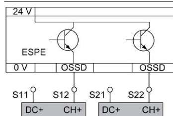
OSSD-Signale
