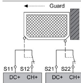
OSSD-Signale
