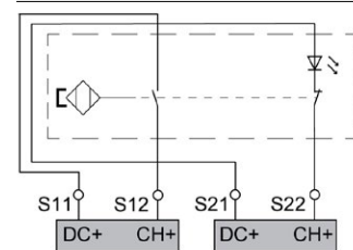
Codierte Magnetschalter
