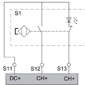
OSSD-Signale
