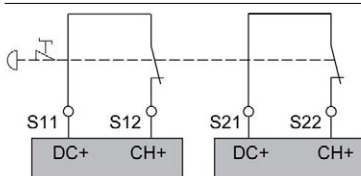
Not-Halt
