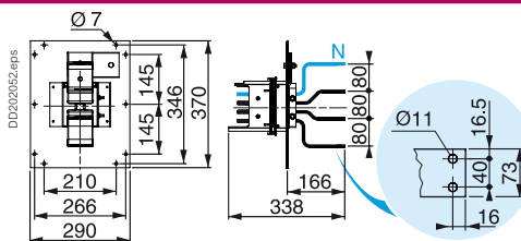
KSA630AE4
