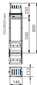
KSA●●●ED4081
