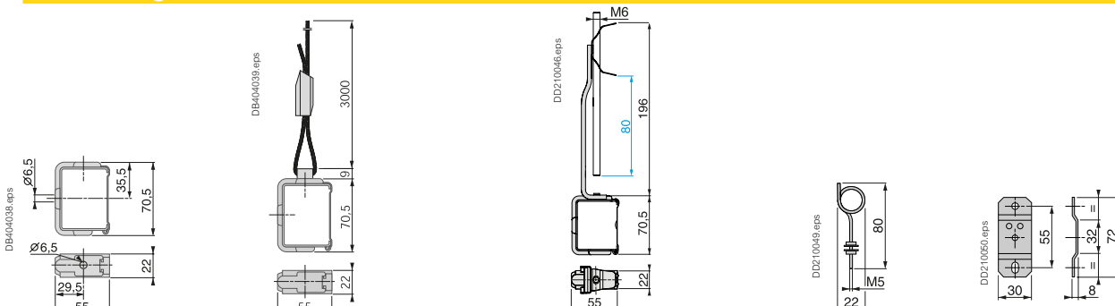
KBA40ZFUW
