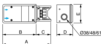
KNT...AB4
