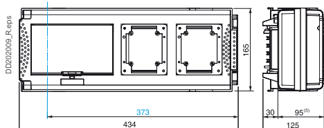
KNB32CP
