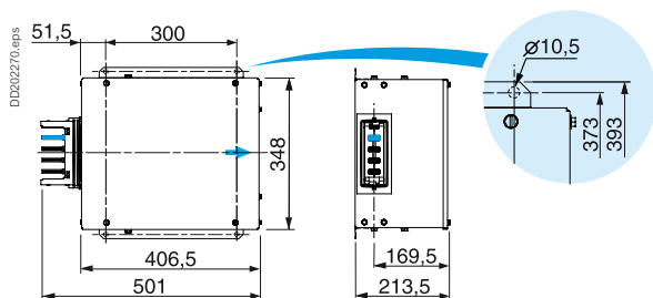
KSA400AB4
