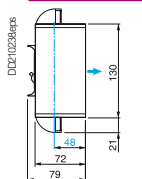
KNB16CM2 KNB16CM2H
