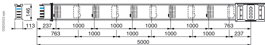
KSA●●●ED45010
