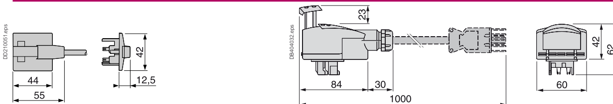
KBC10DCS●01
