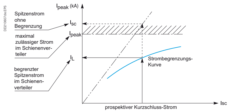
Prüfung der Festigkeit des Schienenverteilersystems gegenüber Spitzenströmen.
