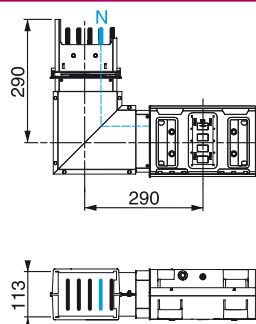
KSA630DLE40
