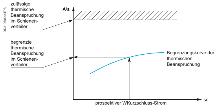
Prüfung der Festigkeit des Schienenverteilersystems gegenüber thermischer Beanspruchung.
