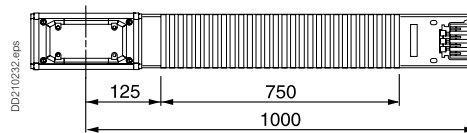
KNA●●●DF410, KNT●●●DF410
