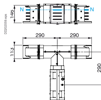
KSA630DTC40
