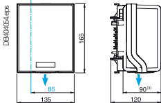
KNB16CN5
