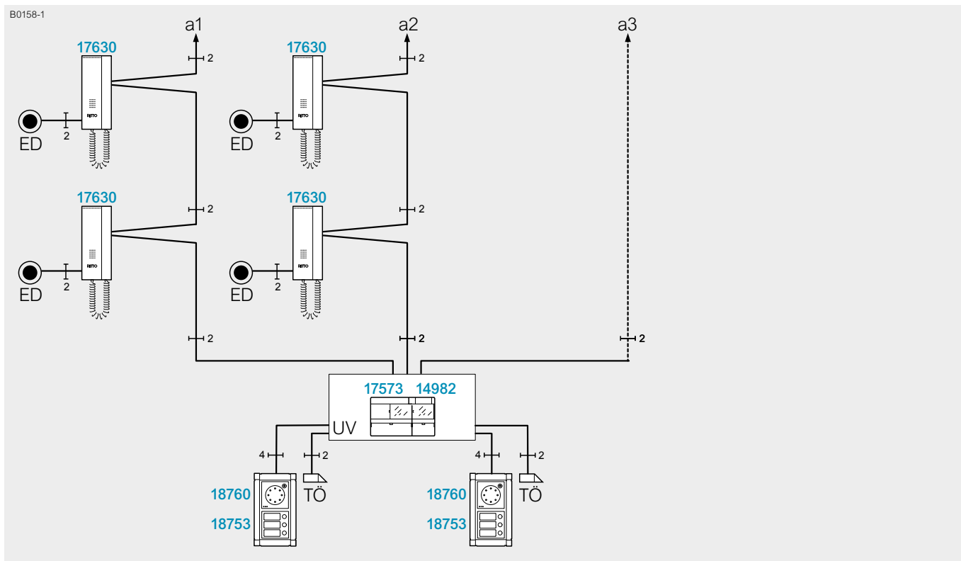
Türumschaltung Artikel-Nr. 14982
