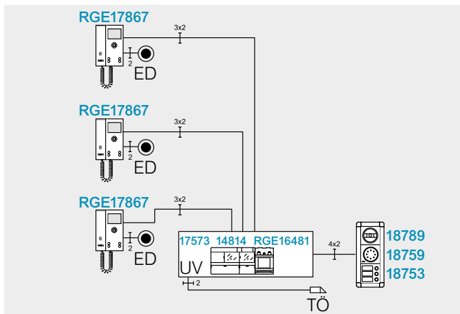
Video-Türsprechanlage mit Linienschalter (sternförmige Verdrahtung)
