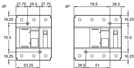
Montageplatte
