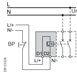
iMN/iMNs mit separater Stromversorgung
