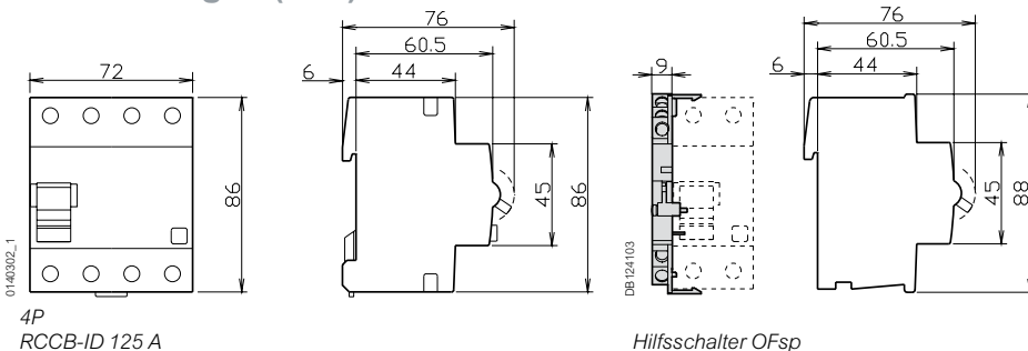
Hilfsschalter OFsp
