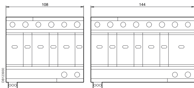
3P PRD1 25r
