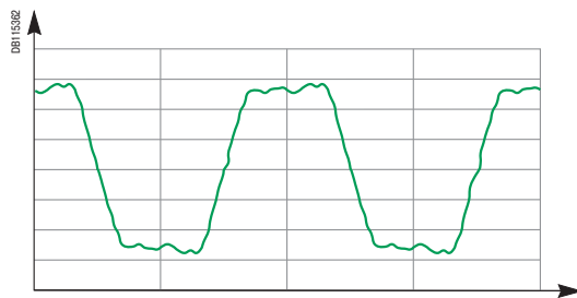
Кривая тока с гармониками
