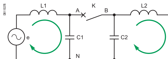
При размыкании K напряжения VAN и VBN находятся в противофазе, что приводит к их взаимному подавлению. Дуга будет повторно возникать до тех пор, пока энергия на ее поддержание не будет израсходована и увеличивающееся расстояние между контактами не прекратит этот процесс
