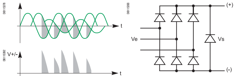
Влияние дисбаланса напряжений на тиристорные устройства
