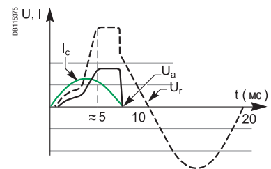
Перенапряжение на клеммах автоматического выключателя с токоограничением.
