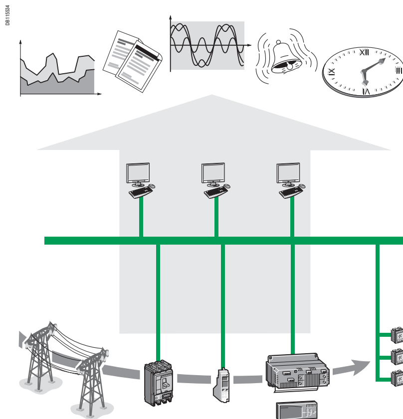
Система управления измерением мощности
