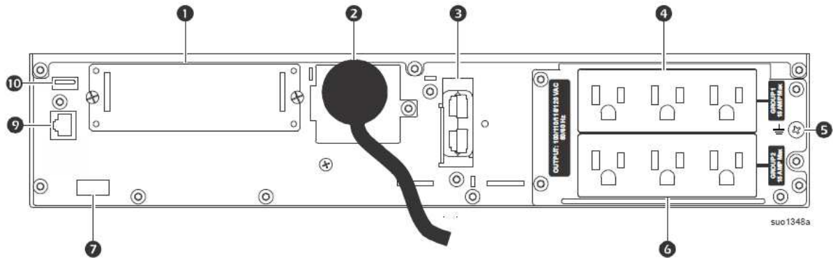
背面パネル
