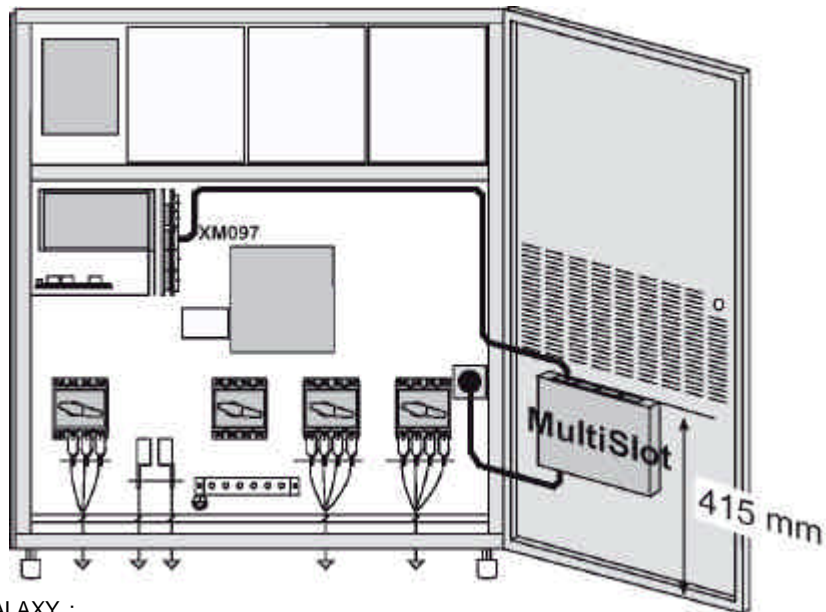
Fig. 3 - GALAXY :
