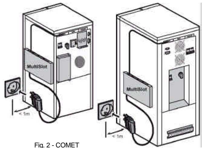
Fig. 2 - COMET
