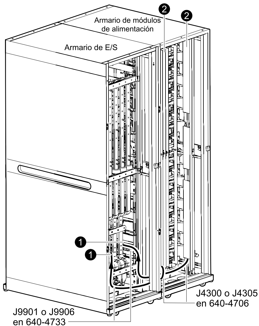
Vista posterior del armario de E/S y el armario de módulos de alimentación
