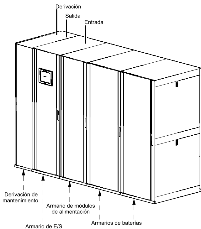
Sistemas con entrada por la parte superior con baterías alineadas en fila
