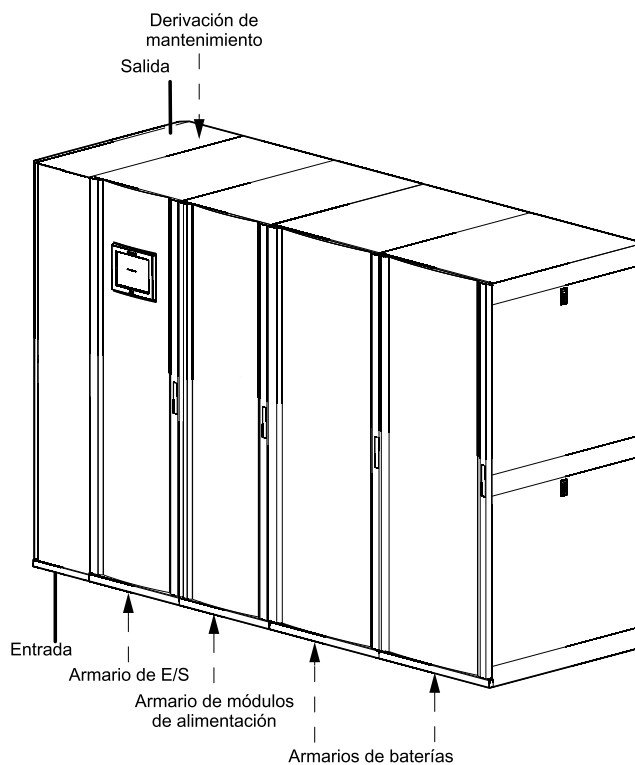
Entrada de cables por la parte inferior con armarios de baterías alineadas en fila
