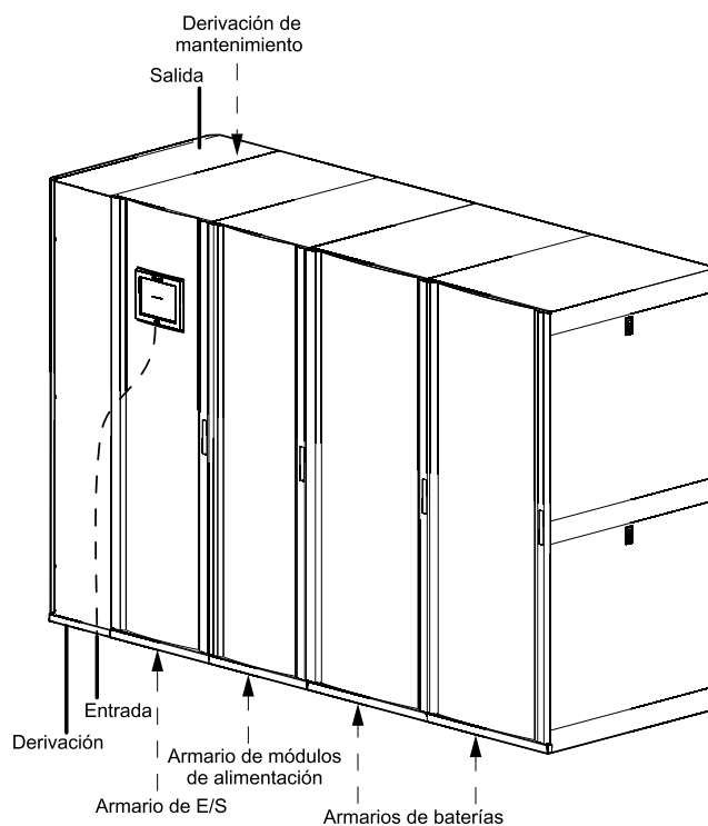
Sistemas de < 250 kW con entrada por la parte inferior con baterías alineadas en fila
