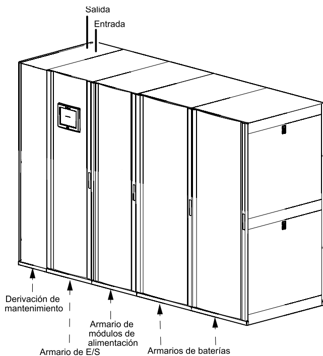
Entrada de cables por la parte superior con armarios de baterías alineadas en fila
