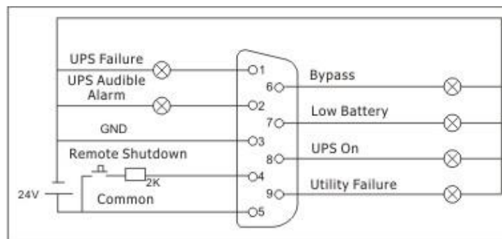
Interfaz de usuario para 24 V
