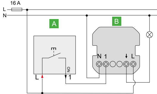
Egypólusú nyomó Wiser intelligens kapcsoló (SDDxxx388)
