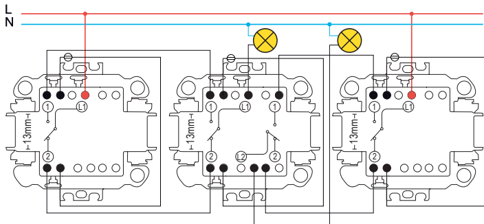
Kettős váltókapcsolás
