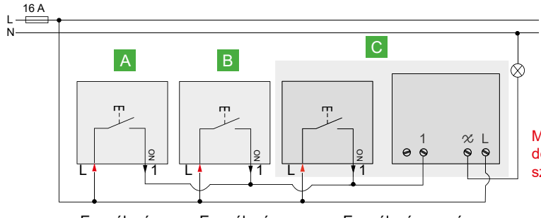
Egypólusú nyomó Egypólusú nyomó Egypólusú nyomó + Wiser fényerőszabályzó mikromodul (CCT5010-0002)
