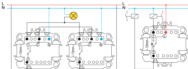
Váltókapcsolás ellenőrzőfényrel
