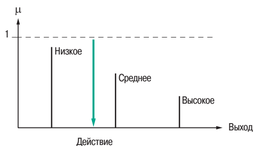
Рис. 32. Дефазификация функции принадлежности одноэлементного множества
