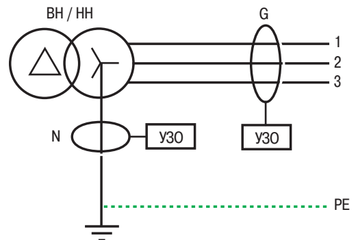
Рис. 16: тор N выдает ту же информацию, что и тор G.
