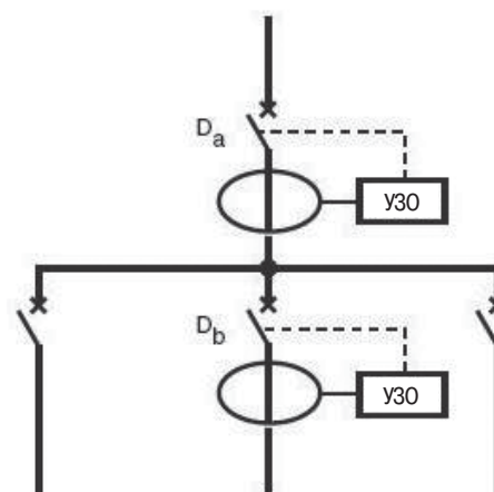
Рис. 20: вертикальная селективность.
