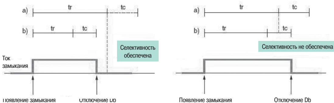
Рис. 21: замедление вышерасположенного УЗО (a) должно учитывать время запаздывания и время отключения нижерасположенного УЗО (b)
