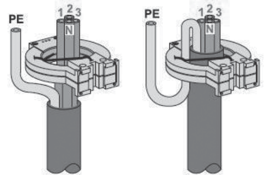
Рис. 14: монтаж торов на кабелях с PE.
