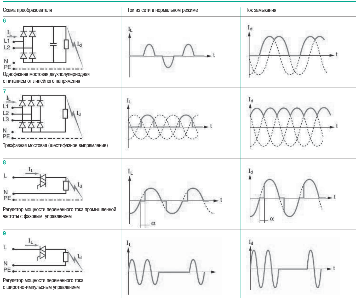
Рис. 33 (продолжение предыдущей страницы): ток замыкания в различных схемах полупроводниковых преобразователей.
