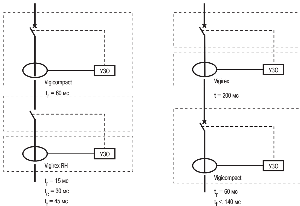
Рис. 22: два примера временной селективности для сочетаний дифференциального автомата типа Vigicomact и реле Vigirex фирмы Merlin Gerin. Следует отметить, что эти времена значительно ниже допустимых времен, приведенных на рис.9.
