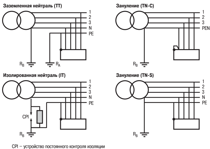
Рис. 6: Три принципиальные схемы заземления – ТТ, TN, IT, установленные стандартом МЭК 60364-1. TN может быть либо TN-C (нейтраль и PE совмещены), либо TN-S (нейтраль и PE разделены).
