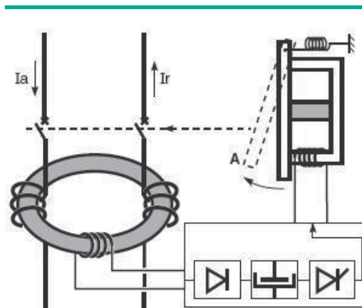
Рис. 11: через посредство тора ток замыкания передает энергию сигнала электромагниту, якорь которого удерживается в притянутом состоянии с помощью постоянного магнита. Когда порог срабатывания достигнут, электромагнит нейтрализует силу притяжения постоянного магнита, якорь под действием пружины отходит от сердечника, приводит в движение контакты – выключатель отключается.
