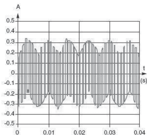
Рис. 35: ток замыкания на выходе трехфазного преобразователя частоты
