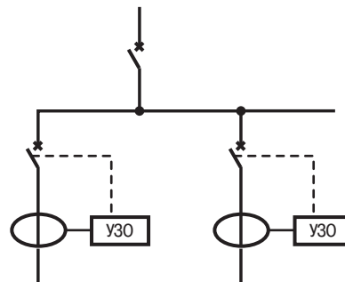
Рис. 23: пример горизонтальной селективности
