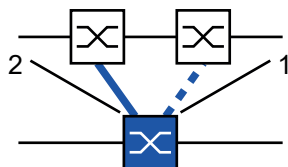
Abb. 57: 1-Switch-Kopplung 1: Kopplungs-Port 2: Partner-Kopplungs-Port
