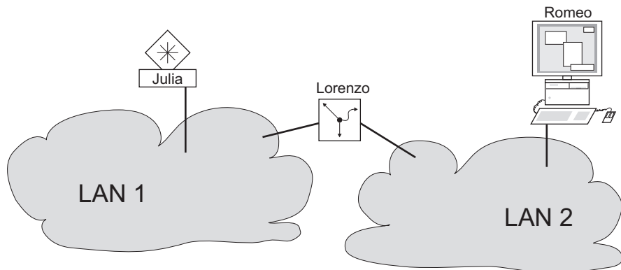
Abb. 14: Management-Agent durch Router von der Netz-Management-Station getrennt
