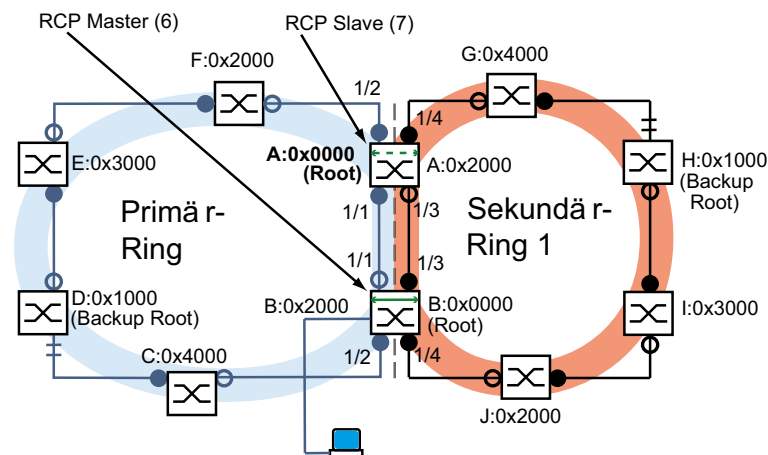
Abb. 69: Primär-Ring mit einem angekoppelten Sekundär-Ring, mit Port-Nummern und RCP-Rollen 6: RCP-Master 7: RCP-Slave
