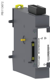
4-Wire RS-485 Option Module
