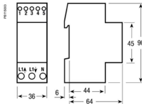
iEM2110/iEM2135/iEM2150/iEM2155 dimensions
