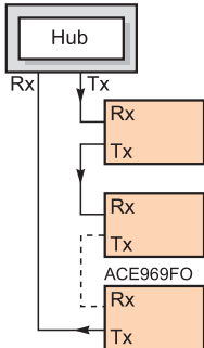
Raccordement en anneau
