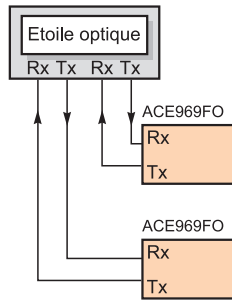
Raccordement en étoile optique
