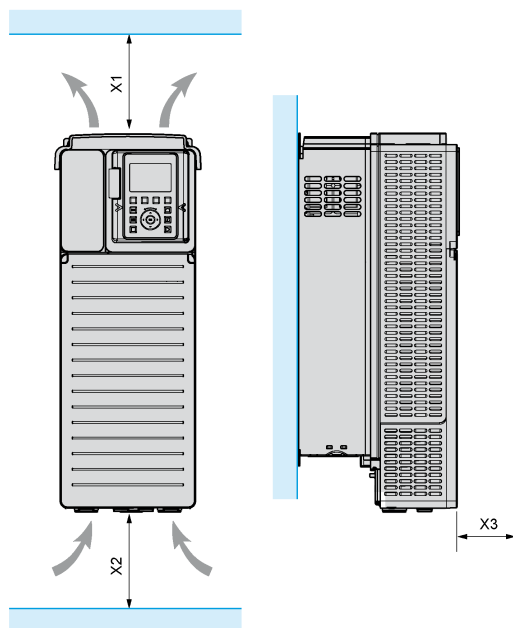
Dégagement minimum en fonction de la taille du variateur
