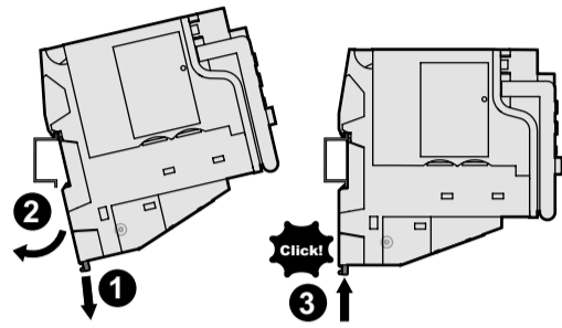
Installing the HU250 module on DIN rail
