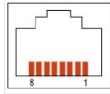
Serielle Modbus- Pinbelegung
