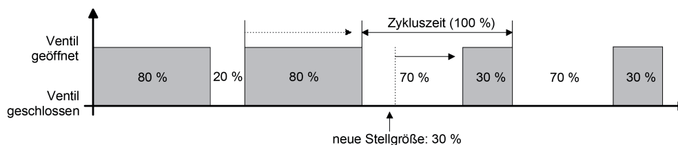
Bild 11: Beispiel einer Stellgrößenänderung 80 % -> 30 % während Schließphase des Ventils
