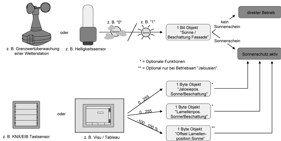
Bild 23: Prinzipialschaltbild des einfachen Sonnenschutzes
