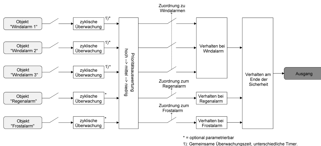
Bild 21: Funktionsschaltbild der Sicherheitsfunktion
