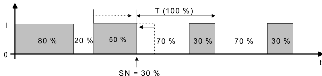
Bild 45: Stellgrößenänderung z. B. von 80 % auf 30 % während Öffnungsphase des Ventils (Öffnungsphase zu lang)
