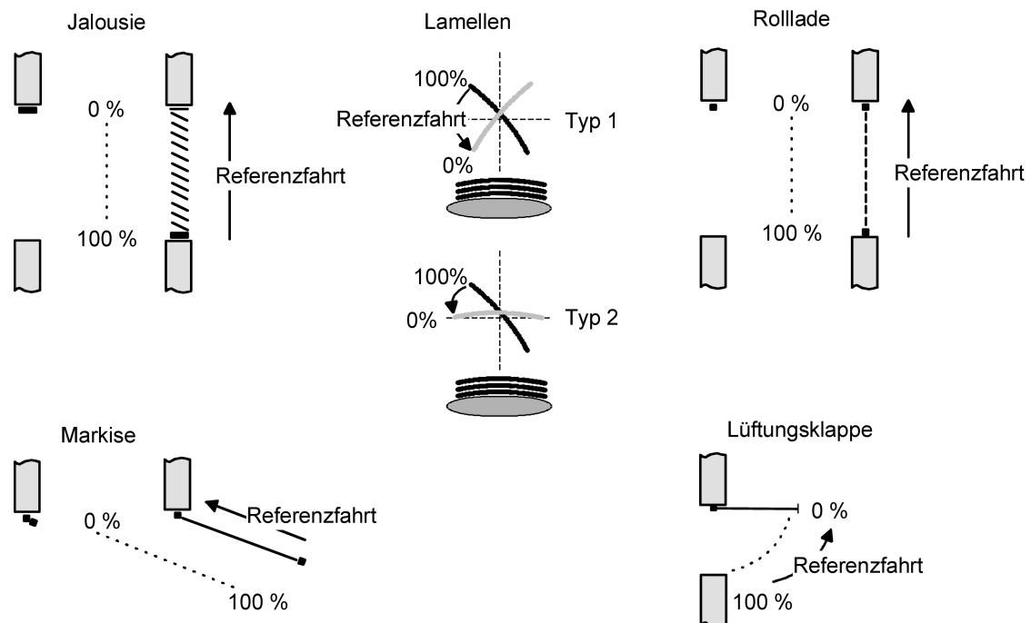
Bild 20: Referenzfahrt
