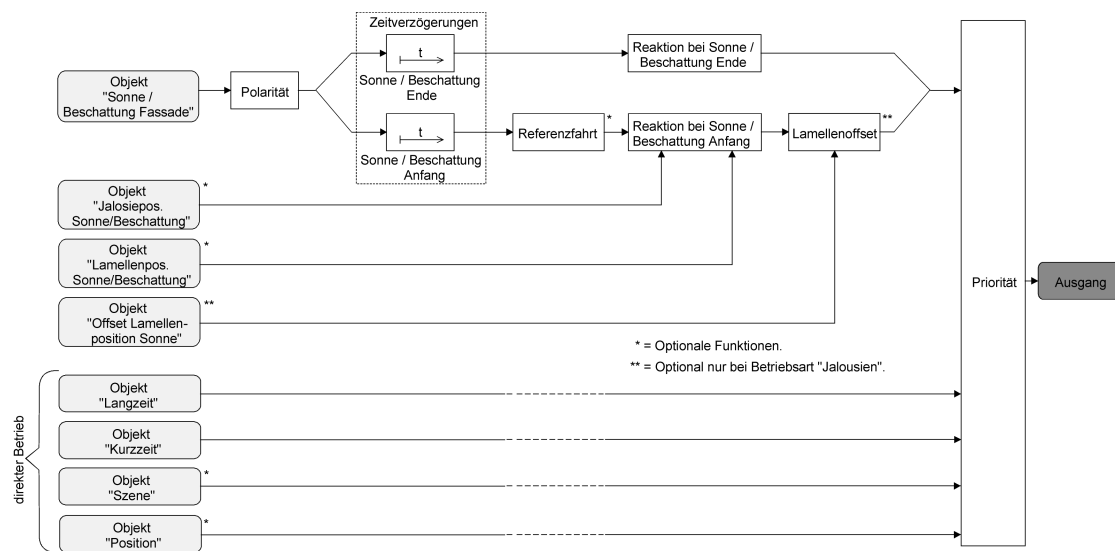
Bild 24: Funktionsschaltbild des einfachen Sonnenschutzes
