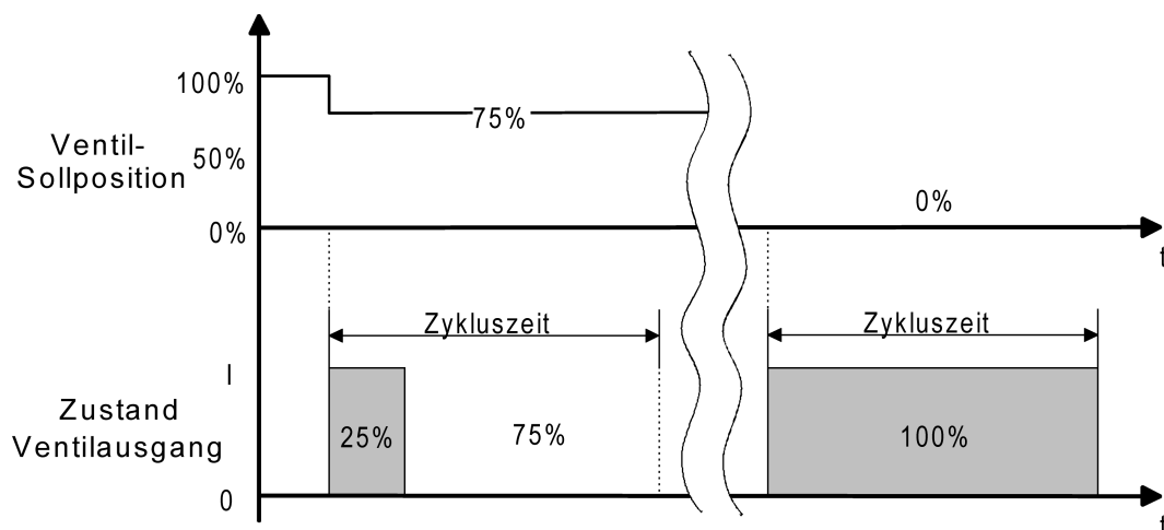
Bild 39: Umsetzung einer stetigen Ventil-Sollposition in ein Ausgangssignal bei stromlos geöffneten Ventilantrieben (Beispiel)
