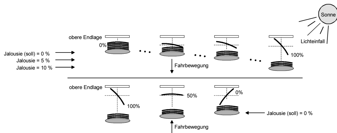
Bild 19: Beispiel für Lamellenpositionierung bei Jalousieposition in der oberen Endlage (Beispielhaft für Lamellentyp 1.)
