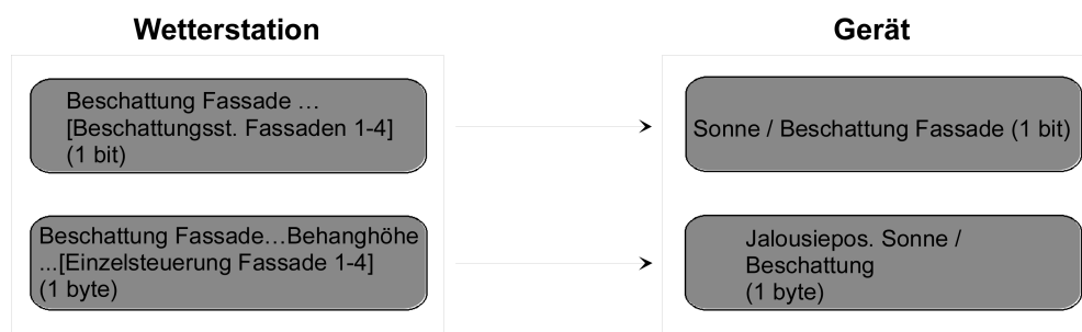
Bild 32: Projektierung der Kommunikationsobjekte für Anwendungsbeispiel V.
