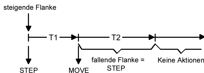
Bild 9: Bedienkonzept "Kurz - Lang - Kurz" bei interner Wirkung der Eingänge 1 und 2
