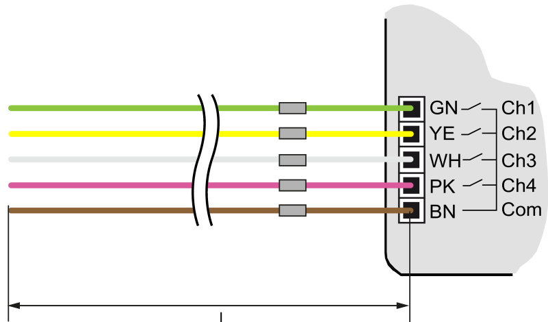
Bild 4: Maximale Leitungslänge
