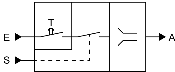
Bild 25: Sperrglied (Filtern / Zeit)
