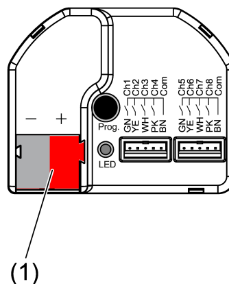
Bild 3: Busanschluss
