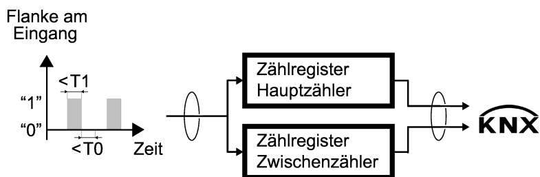
Bild 13: Funktionsschema des Impulszählers
