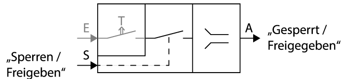
Bild 22: Schematische Darstellung "Sperrfunktion"
