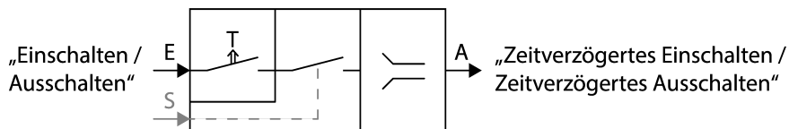
Bild 20: Schematische Darstellung "Zeitverzögert Ein- und Ausschalten"
