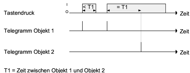
Bild 12: Beispiel zum Bedienkonzept "Objekt 1 und Objekt 2"
