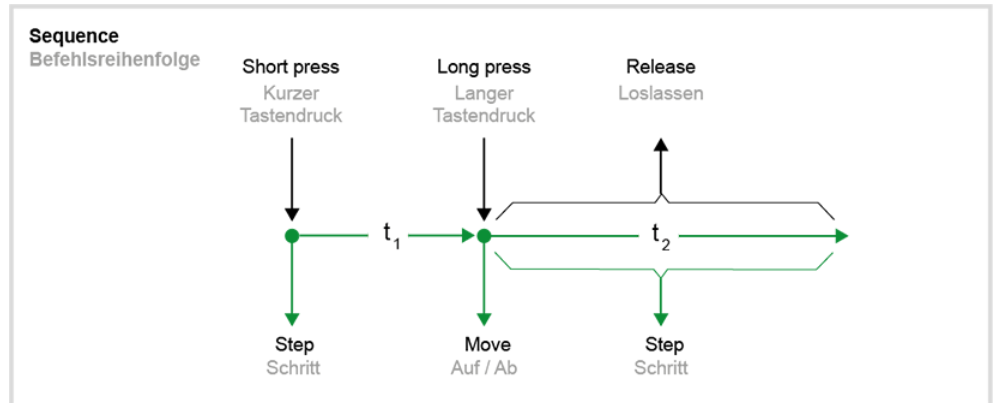
Bild 7: Bedienkonzept "Schritt-Auf/Ab-Schritt"
