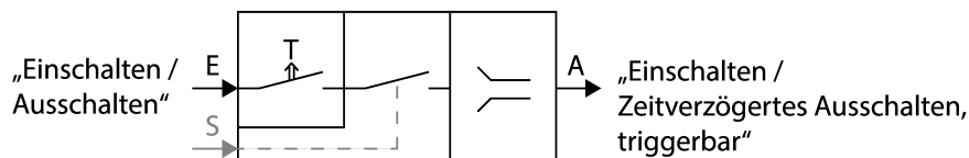
Bild 21: Schematische Darstellung "Treppenhausfunktion"
