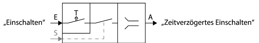
Bild 18: Schematische Darstellung "Zeitverzögert Einschalten"
