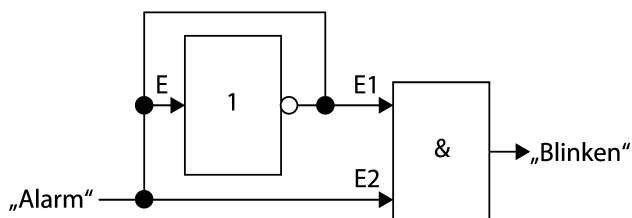
Bild 17: Schematische Darstellung "Blinken"
