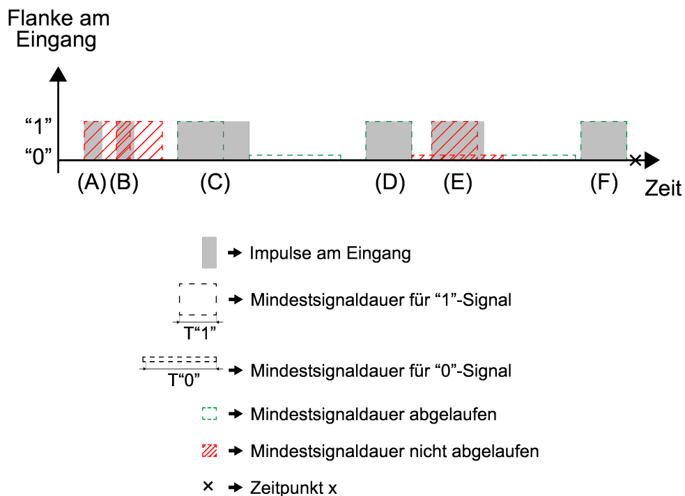
Bild 16: Beispiel zur Einstellung der Mindestsignaldauer
