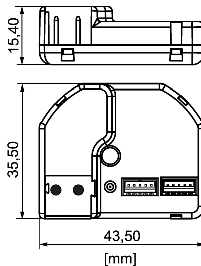
Bild 2: Maßzeichnung
