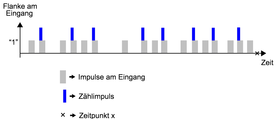
Bild 15: Beispiel zur Einstellung der Zählerstandsänderung pro Zählimpuls
