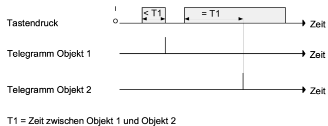
Bild 15: Beispiel zum Bedienkonzept "Objekt 1 oder Objekt 2"
