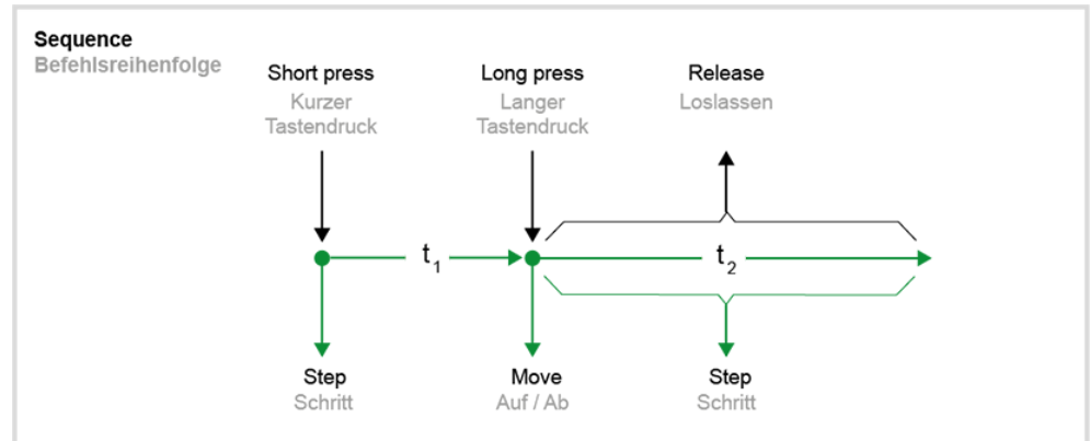
Bild 11: Bedienkonzept "Schritt-Auf/Ab-Schritt"
