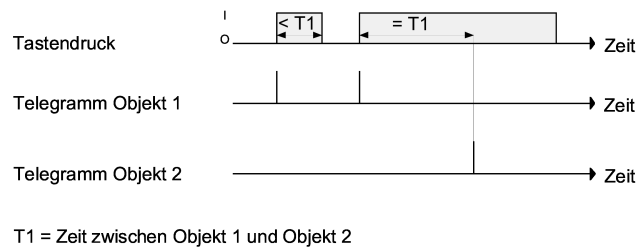
Bild 16: Beispiel zum Bedienkonzept "Objekt 1 und Objekt 2"
