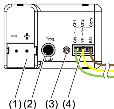
Bild 1: Gerätevariante 2fach
