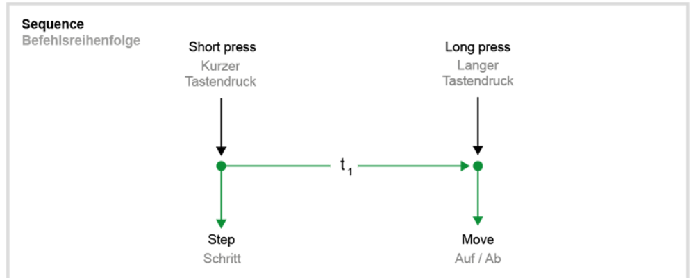
Bild 13: Bedienkonzept "Schritt - Auf/Ab"
