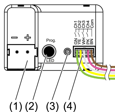
Bild 2: Gerätevariante 4fach
