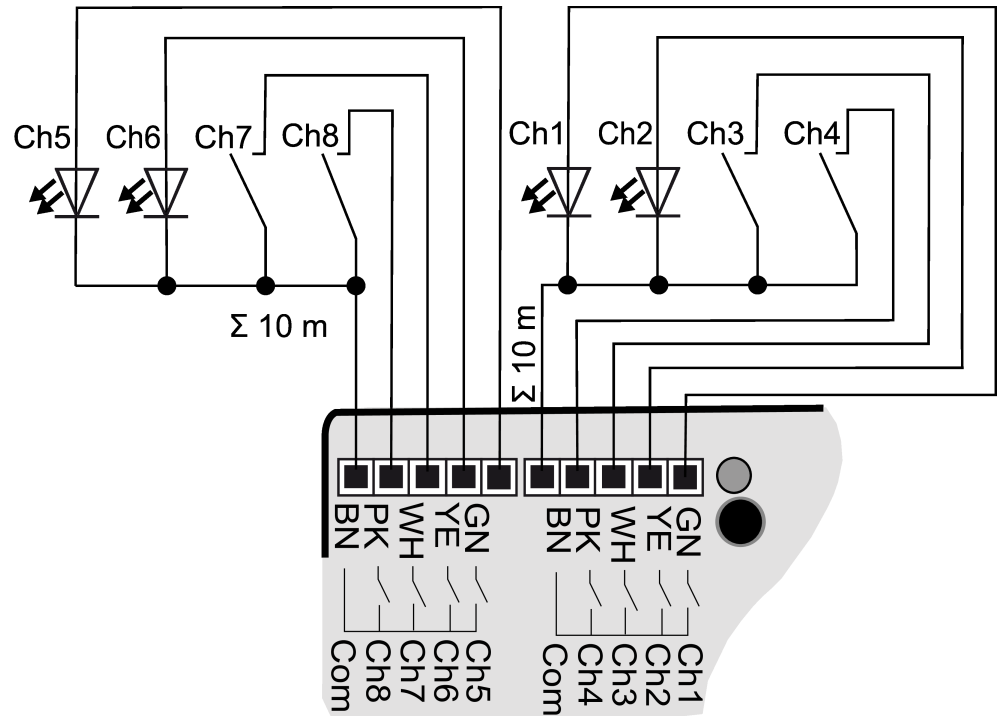
Bild 9: Anschlussbeispiel Tasterschnittstelle 8fach
