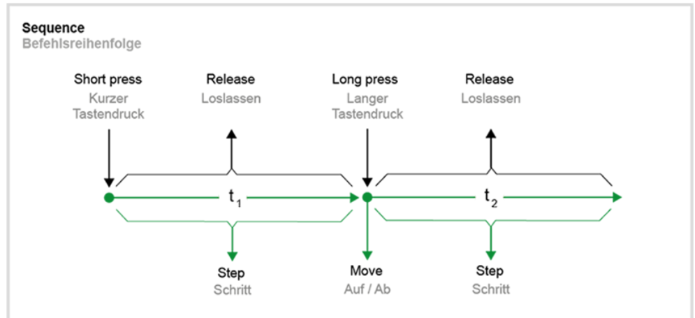
Bild 14: Bedienkonzept "Auf/Ab – Schritt oder Schritt"
