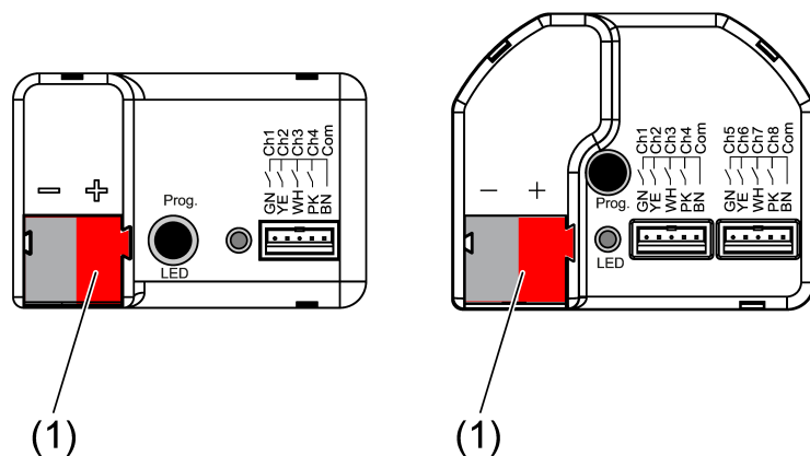
Bild 5: Busanschluss
