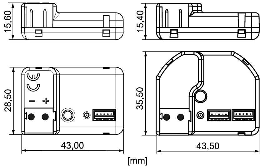
Bild 4: Maßzeichnung
