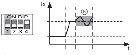
(B) Commande rapide de la lumière
