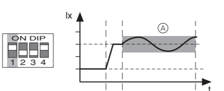
(A) Commande lente de la lumière
