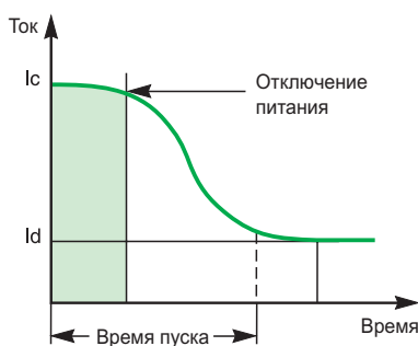
Категория применения AC4: контактор должен отключать пусковой ток двигателя
