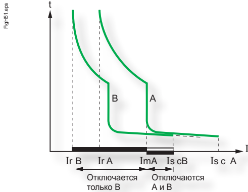
Частичная селективность автоматических выключателей A и B
