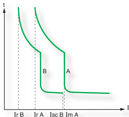
Полная селективность автоматических выключателей А и В
