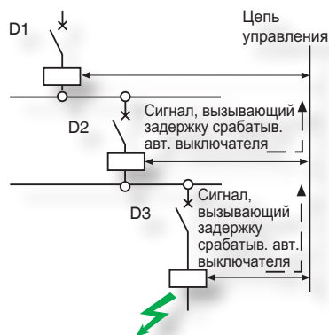
Логическая селективность
