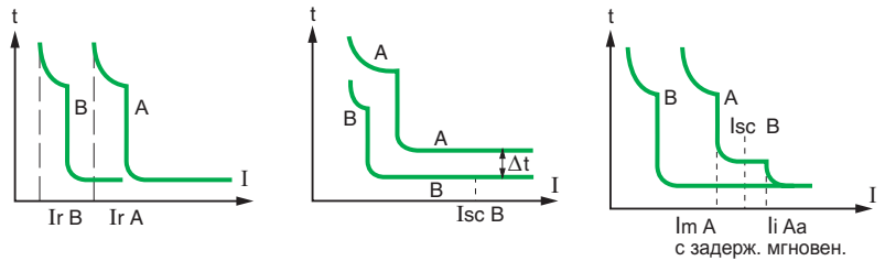
Токовая селективность
